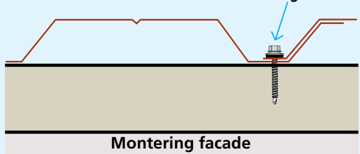
Monteringsskrue
