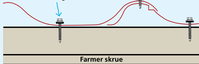
Monteringsskrue
