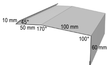
84 Blindfals
