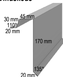
71a Vindskede
