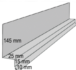
9 Lodret inddækning
