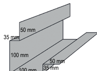
13a Hjørne hatteprofil til VP35 og Sinus 35
