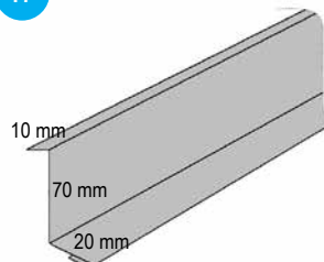
17 Løskant
