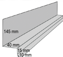
10 Sålbank
