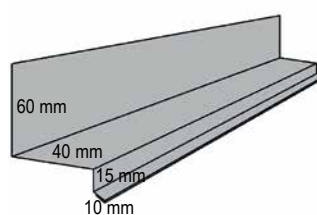
8a Vandnæse sokkel til VP35 og Sinus 35
