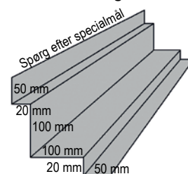
14b Indv. hatteprofil til VP20 og Sinus 18
