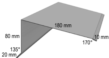
77 Pulttagsrygning
