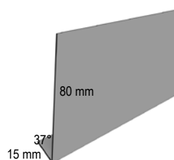
83 Bundprofil
