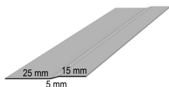
74 Samleprofil
