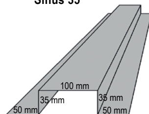
14c Indv. hatteprofil til VP35 og Sinus 35
