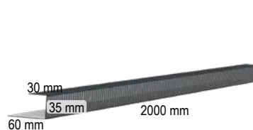
75 Ventilationsliste
