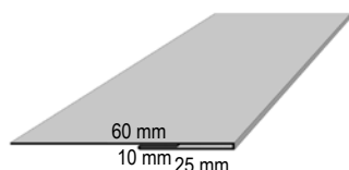
84 Blindfals
