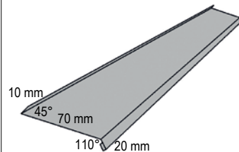
10 Sålbank
