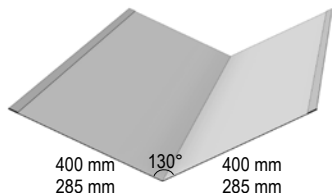
73 Skotrende - enkelt
