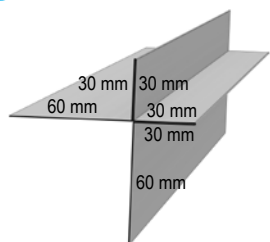
78 Udvendig hjørneprofil
