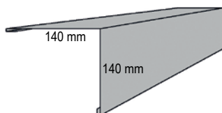
11 Udvendtigt hjørne
