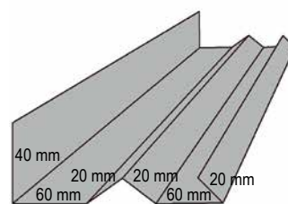
17 Løskant
