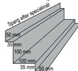
14c Indv. hatteprofil til VP35 og Sinus 35
