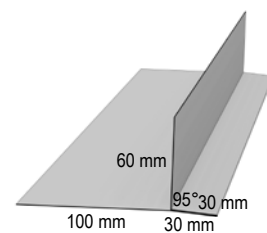
80 Vandret lysningsprofil
