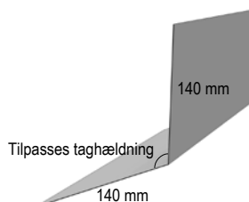
76a Tilslutning til væg
