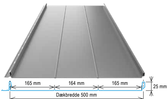
Easy-Clickfals 500-164
