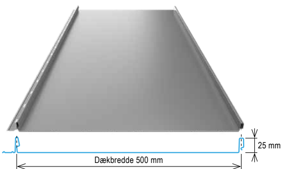
Easy-Clickfals 500-164
